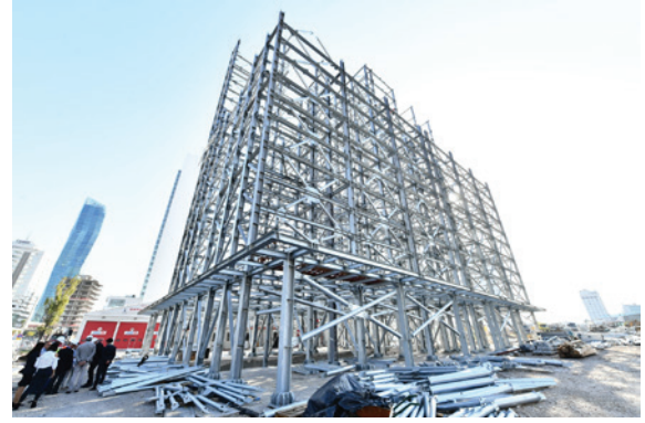
Adliye Tam Otomatik Katlı Otopark
